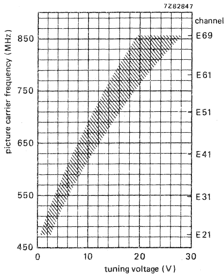
Fig. 10 U.H.F. band.
