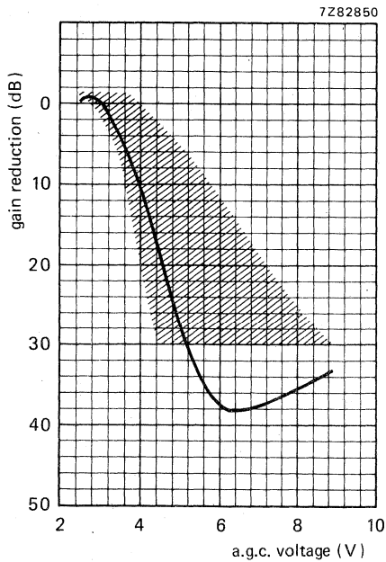
Fig. 7 U.H.F. band.
